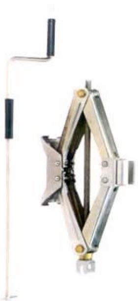
剪式千斤頂
